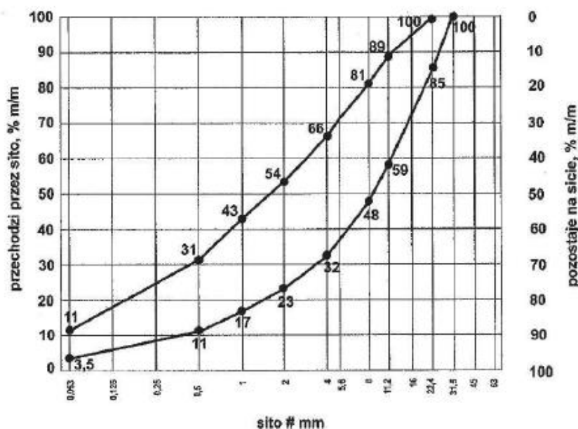
Rys.1.2. Uziarnienie mieszanki CBGM 0/22,4
