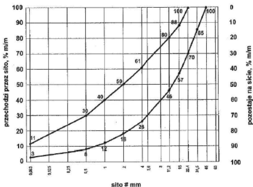
Rys.1.1. Uziarnienie mieszanki CBGM 0/31,5
