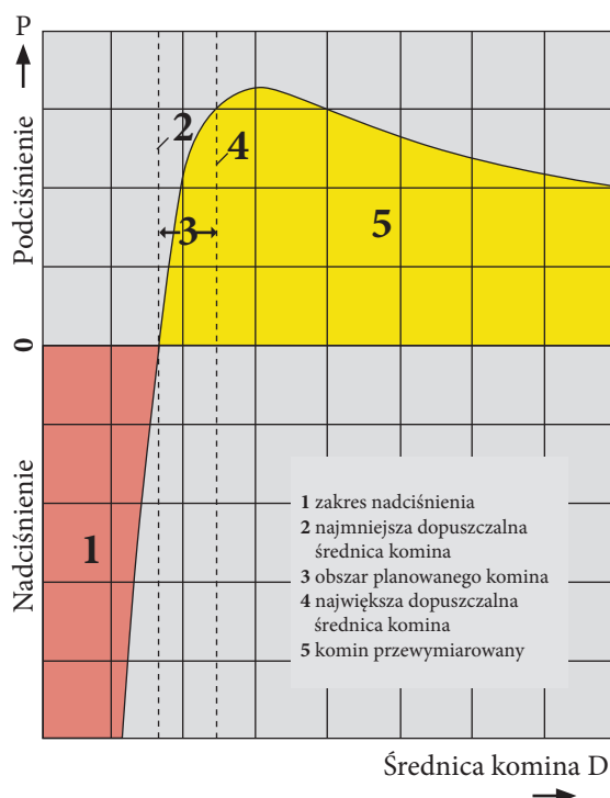
Rys. 30. Doboru rozmiaru kominą dla warunków panujących w przewodzie kominowym, z ciągiem naturalnym.
