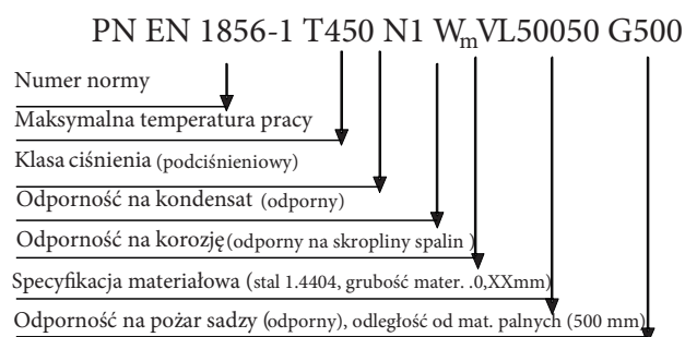
Rys. 32. Sposób znakowania elementów wkładu kominowego
