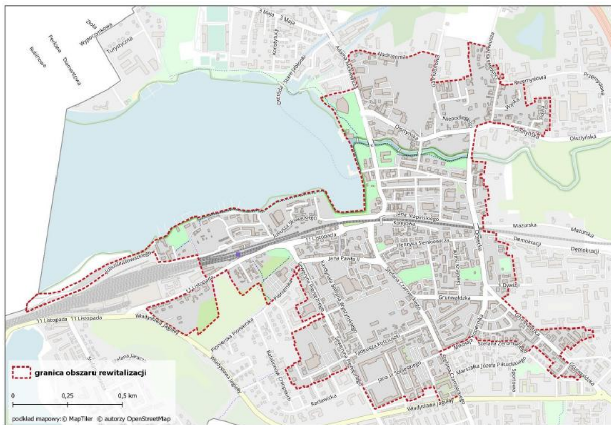
Rys. 9. Obszar rewitalizacji
